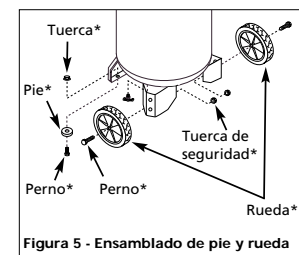
Figura 5 - Ensamblado de pie y rueda
