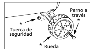
Figura 3 - Para ensamblar las ruedas
